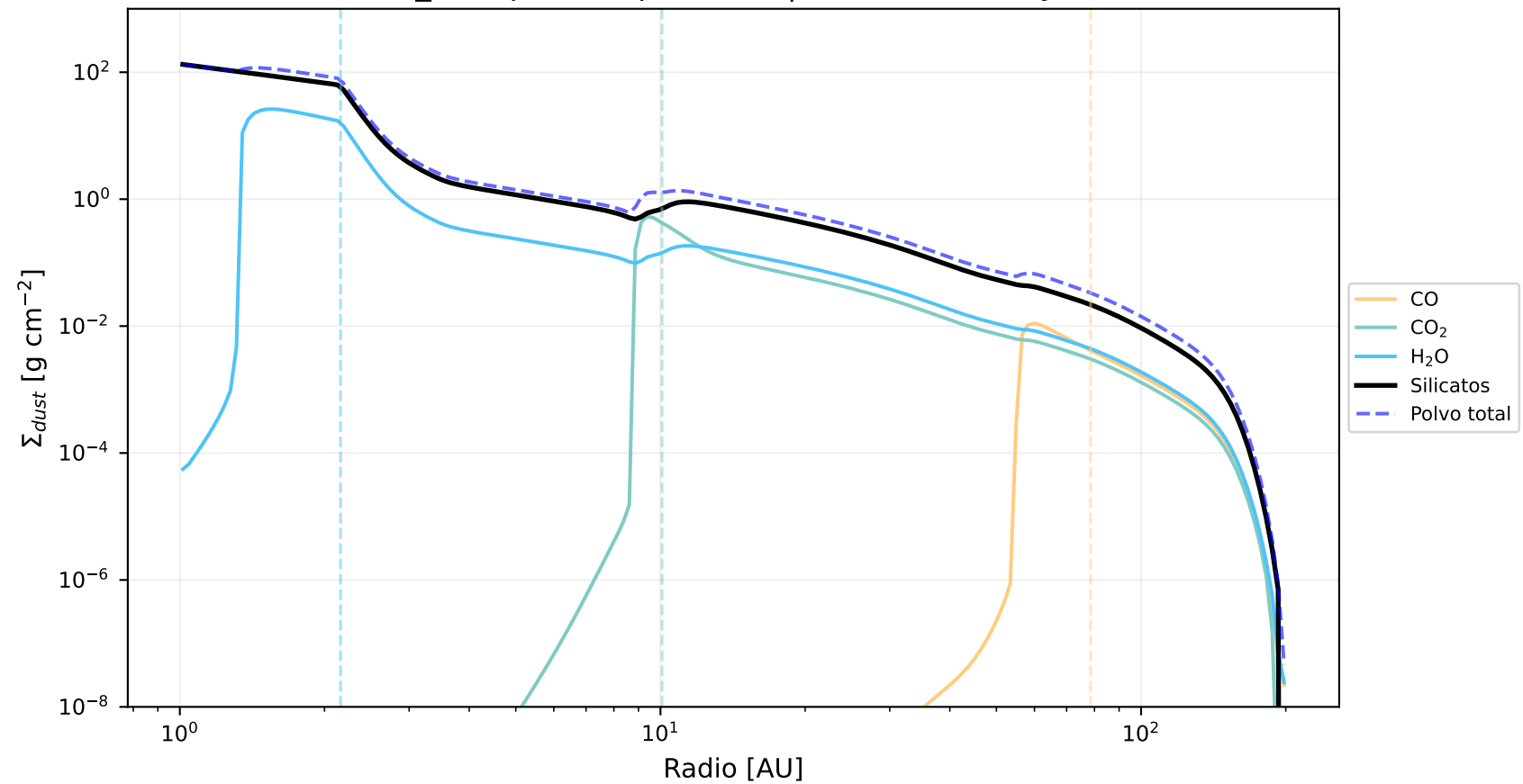
\Sigma_{\text{dust}} por componente | t = 1.00\text{e}+05 yr
